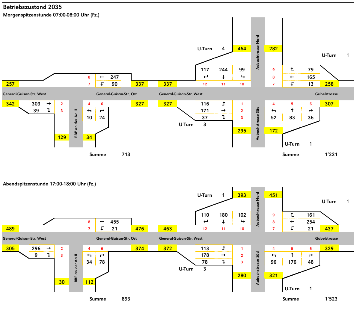
Abbildung 17: Verkehrsmenge Betriebszustand 2035
